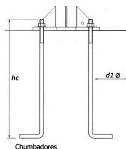
Chumbadores
